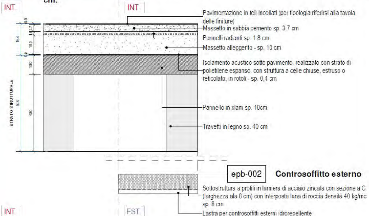
pavimento P1 tipo.JPG
