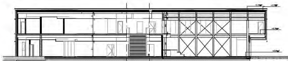
Sezione CC' Scala 1:100
