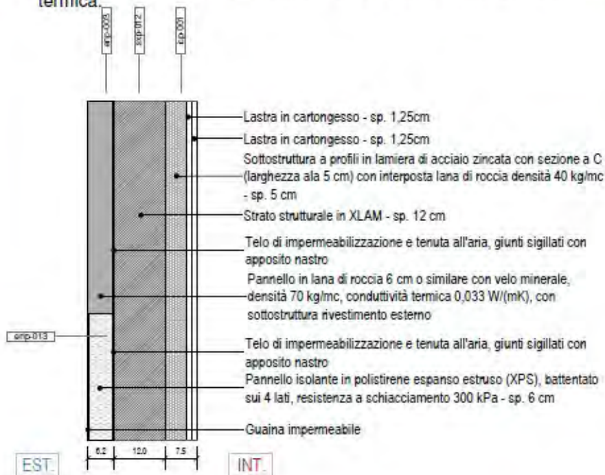
parete perimetrale tipo.JPG
