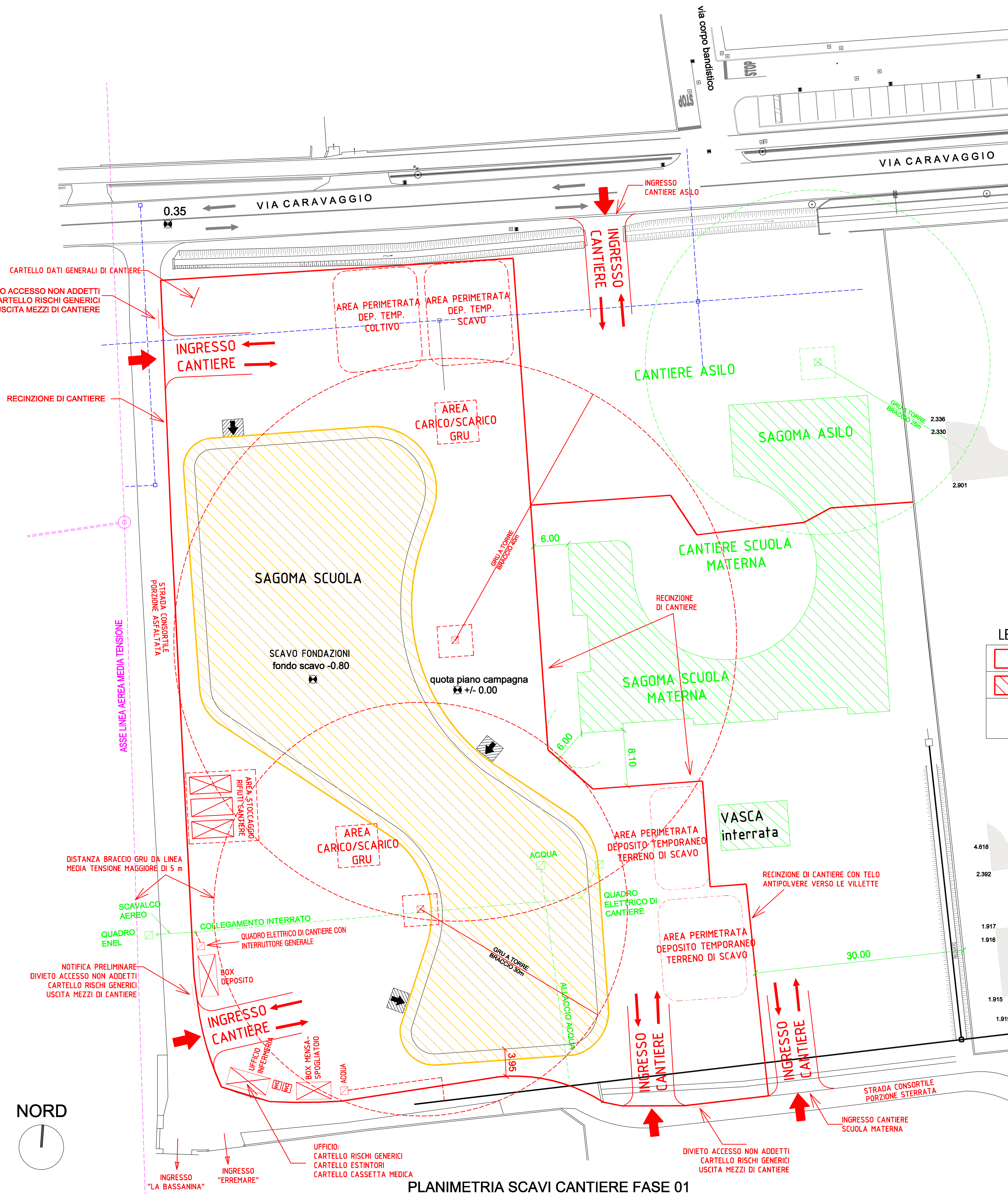
PLANIMETRIA SCAVI CANTIERE FASE 01
