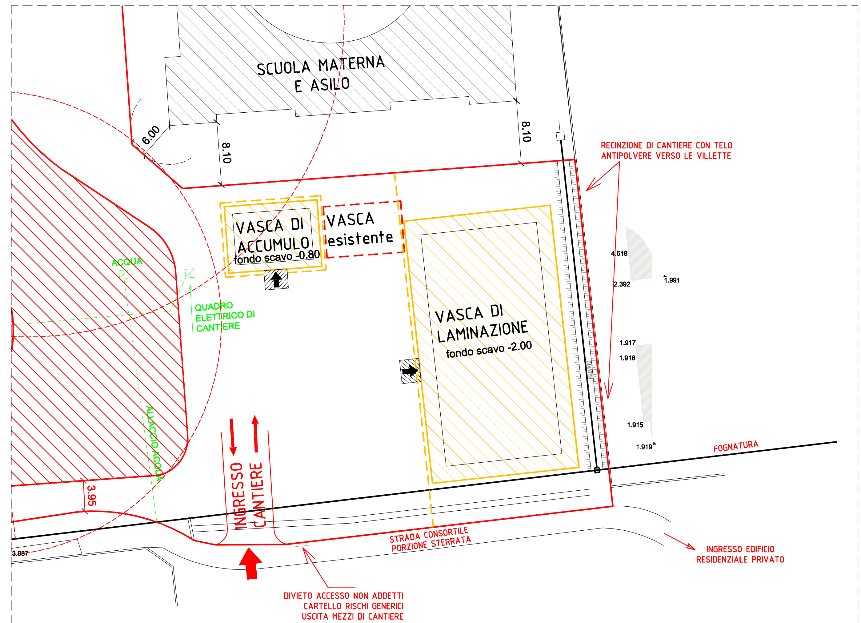
PLANIMETRIA SCAVI CANTIERE FASE 02
